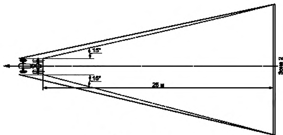
Рисунок 4.2 — Видимость белого огня сзади
