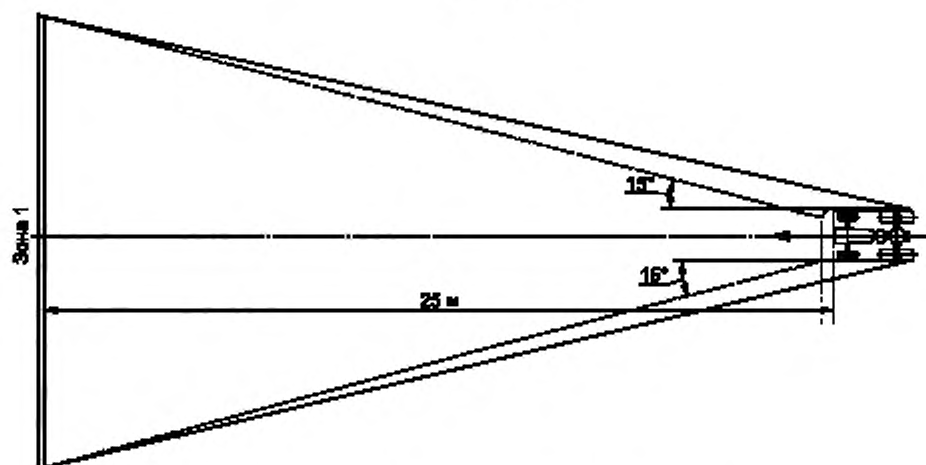
Рисунок 4.1 — Видимость красного огня спереди
