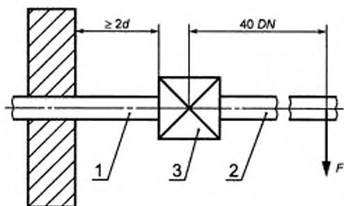
Рисунок 8 — Схема испытания на воздействие изгибающего момента
