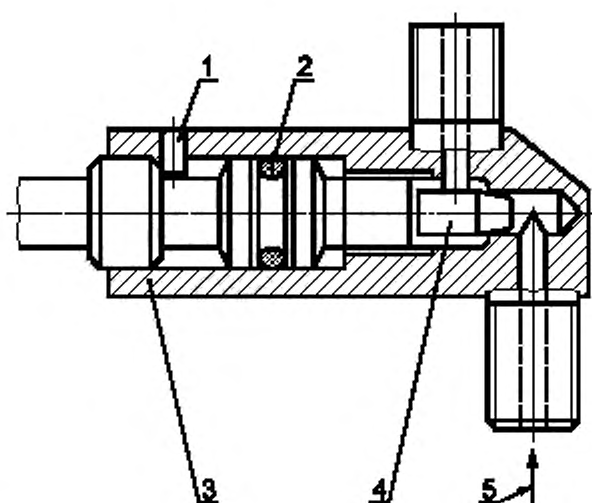
Рисунок 5 — Схема игольчатого крана
