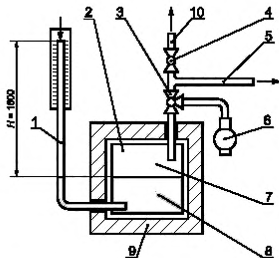
1 — трубка со шкалой в миллиметрах; 2 — термически изолированный сосуд под давлением; 3 — трехходовой кран; 4 — кран; 5 — патрубок для присоединения испытуемого образца; 6 — компрессор; 7 — воздушный объем 1 дм 3 ; 8 — вода; 9 — теплоизоляция; 10 — напорная трубка
