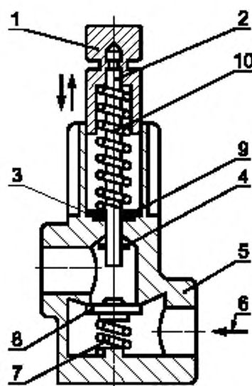
1 — кнопка; 2 — шток; 3 — кольцо уплотнительное; 4 — стопор штока; 5 — корпус крана; 6 — впускное отверстие; 7 — пружина; 8 — тарелка; 9 — шайба; 10 — пружина штока
