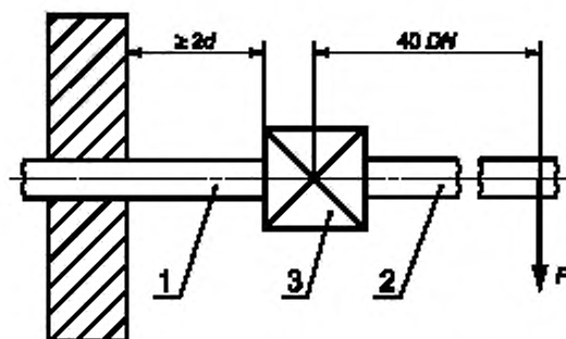
d — внешний диаметр; 1 — первая труба; 2 — вторая труба; 3 — испытуемый клапан
