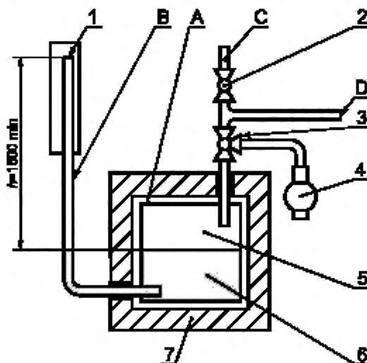
A — теплоизолированный сосуд давления; B — измерительная трубка; C — трубка под давлением; D — соединение с испытываемым клапаном; I — миллиметровая шкала; 2 — вентиль; 3 — трехходовой кран; 4 — компрессор; 5 — воздушная полость объемом 1 дм 3 ; 6 — вода; 7 — теплоизоляция
