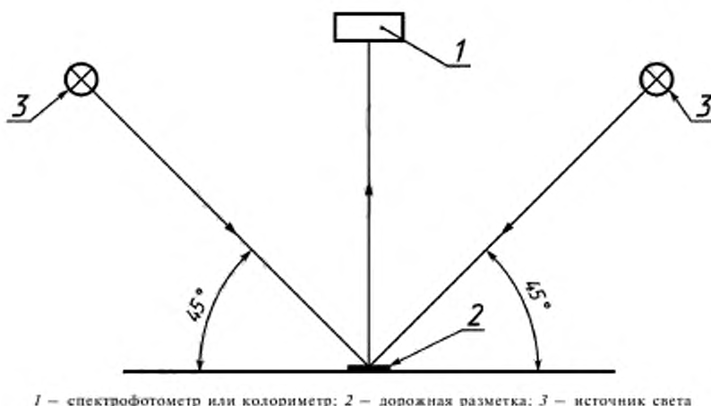
1 — спектрофотометр или колориметр; 2 — дорожная разметка; 3 — источник света Рисунок Г.1 — Схема измерения координат цветности и коэффициента яркости дорожной разметки
