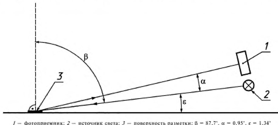
Рисунок Г.2 — Схема измерения коэффициента световозвращения дорожной разметки для условий темного времени суток при освещении фарами автомобиля и сухом покрытии
