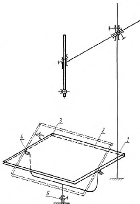
1 — держатель образца; 2 — рамка, прижимающая образец к держателю; 3 — пружина для прижатия рамки к держателю; 4 — подшипник с фиксатором для закрепления держателя в двух крайних положениях (в горизонтальном и под углом 30^\circ ); 5 — подшипник с фиксатором для закрепления держателя в положении поворота на 90^\circ вокруг вертикальной оси
