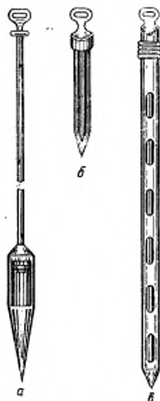
Шупы: а — конусный; б — мешочный; в — цилиндрический
