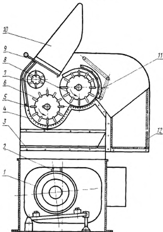
1—электродвигатель; 2—клиноременная передача; 3—сборник сорных примесей; 4—колосниковая решетка; 5—колки; 6—колковый барабан; 7—питающий валок; 8—колковый барабан; 9—заслонка; 10—загрузочный бункер; 11—откидная крышка; 12—ящик для очищенного хлопка-сырца.
