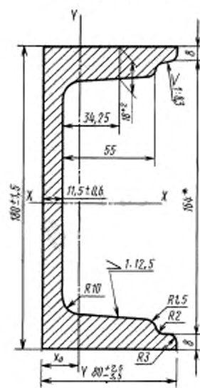
Профиль № 6
