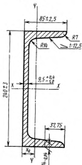
Профиль № 5
