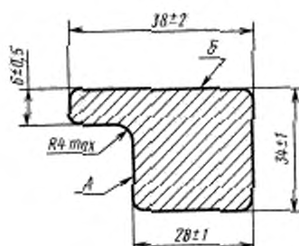
Профиль № 8
