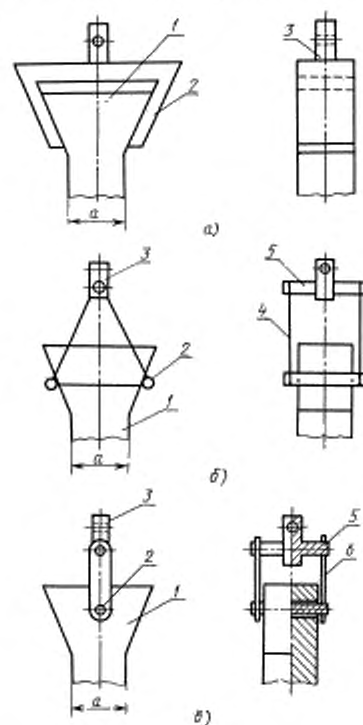
Схема захватов для образца с галтелями
