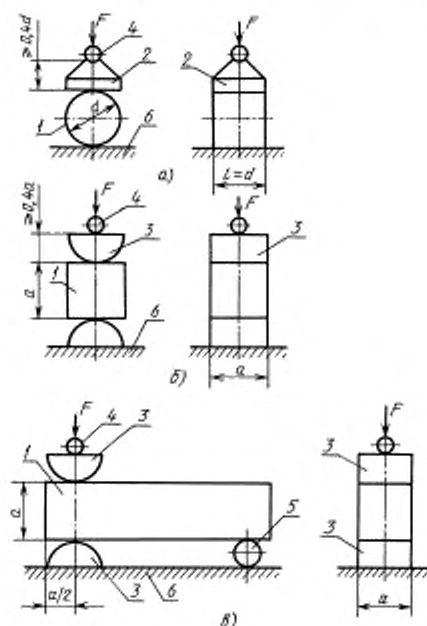
Схема устройств испытаний на растяжение при раскалывании
