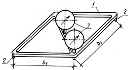
Схема прибора для измерений отклонений от плоскостности
