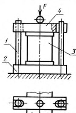
Схема кондуктора
