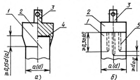
Схема приклеиваемых и анкерных захватов
