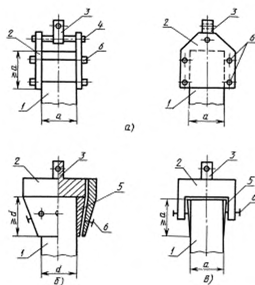
Схемы зажимных захватов
