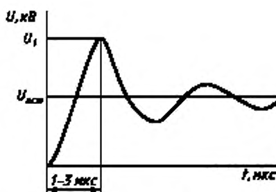
Рисунок Д.2 — Форма грозовых импульсов, характерная для точек присоединения а, в, з на рисунке Д.1.
