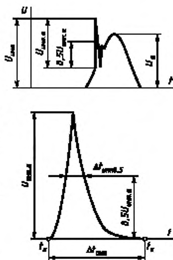
Рисунок Б.3 — Параметры импульсного напряжения
