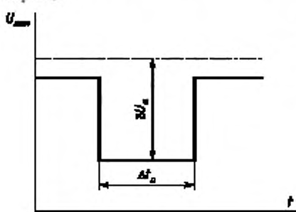
Рисунок Б.2 — Провал напряжения
