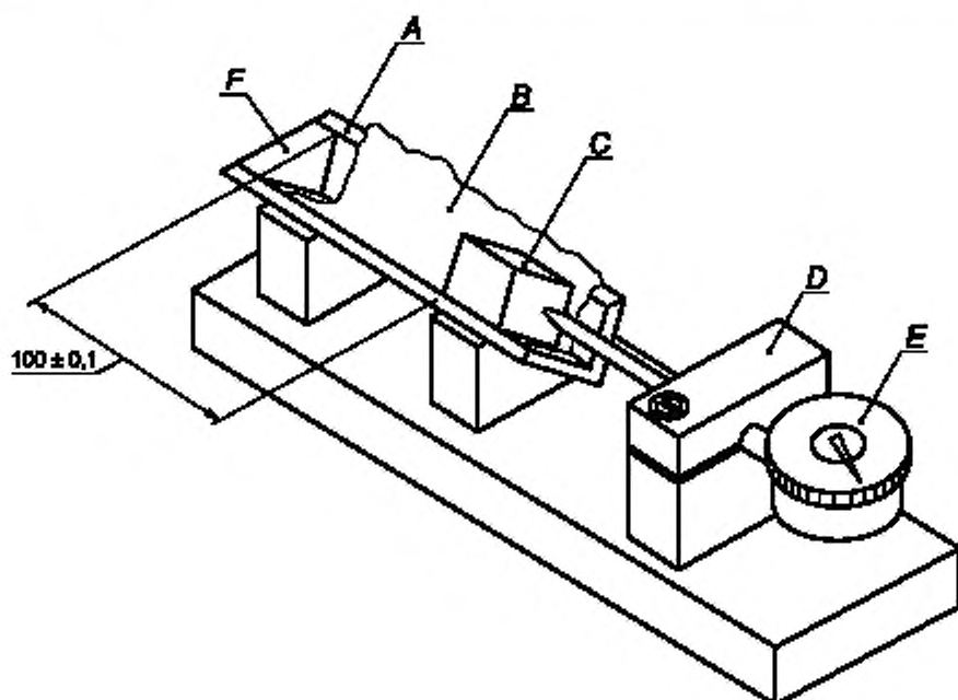
А — желоб; В — лист из фторопласта; С — куб; D — держатель датчика, E — цифровой индикатор или эквивалент; F — неподвижная концевая вставка
