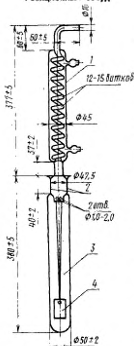
1—холодильник; 2—шпиф; 3—пробирка; 4—пластинка
