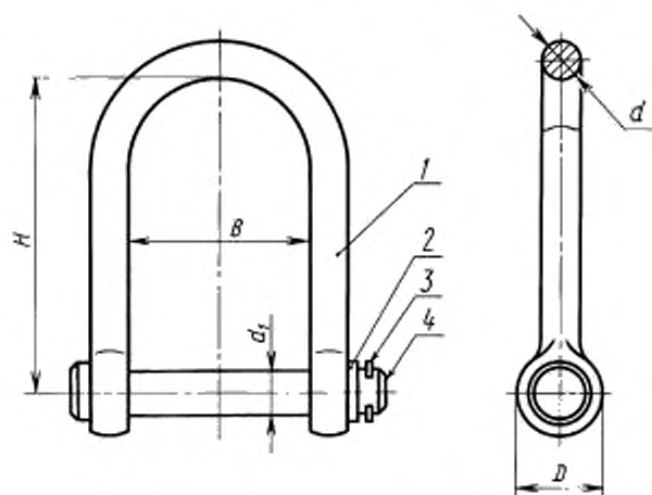
Скоба подвесная
