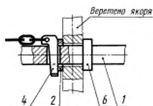
Крепление штока в рабочем положении
