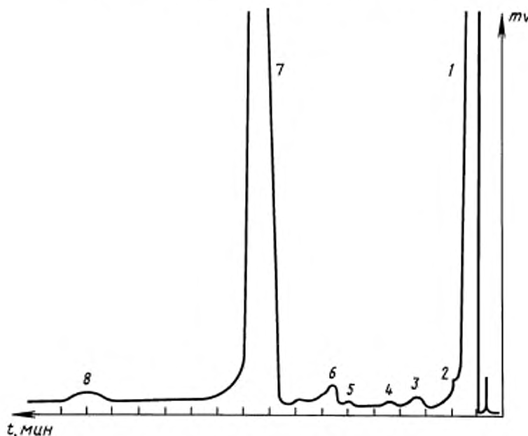
Типовая хроматограмма технического гексахлорэтана
