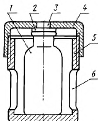
1 — пенициллиновая склянка; 2 — пробка; 3 — отверстие в крышке; 4 — навинчивающаяся металлическая крышка; 5 — корпус металлического стаканчика; 6 — прорез в корпусе стаканчика
