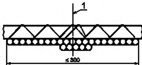
Рисунок 2 — Кабели, закрепленные на передней стороне стандартной лестницы без зазора (комплекты отрезков кабелей находятся в контакте)
