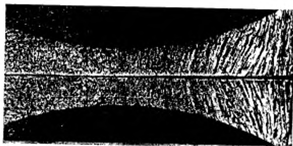
б — слоистый излом в краевой части заготовки
