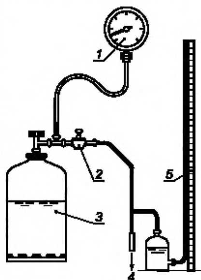
1 и 5 — манометры; 2 — регулятор давления; 3 — баллон со сжиженным газом; 4 — газовому вводу прибора
