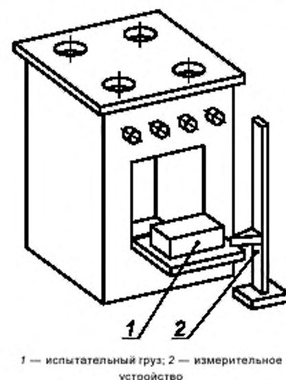
Рисунок 7 — Испытание на прочность дверцы духовки
