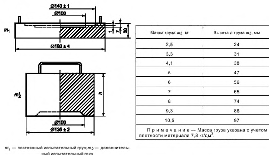
Рисунок 6 — Масса испытательного груза
