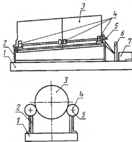
Устройства для перемешивания лакокрасочных материалов
