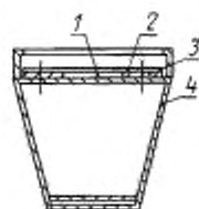
1 — отверстие для ввода пробоотборочной трубки; 2 — нажимная плита; 3 — волокистая шайба; 4 — паяное соединение
