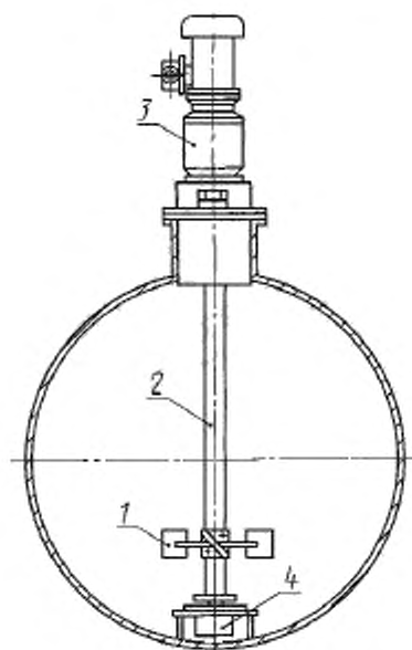
Перемешивающее устройство для цистерн
