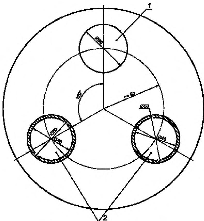
1 — твердый политетрафлюороэтилен; 2 — наполненные цилиндры
