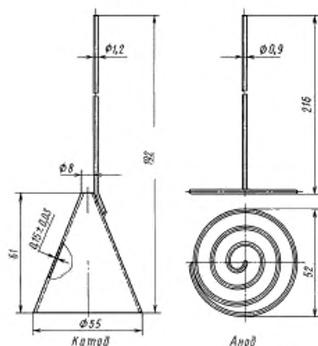
Изделие № 309—1. Масса 19,0 г Изделие № 309—2. Масса 13,0 г
