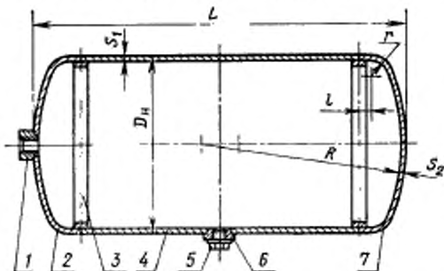
1—штуцер дна; 2—дно с отверстием; 3—кольцо подкладное; 4—обечайка; 5—пробка; 6—штуцер обечайки; 7—дно глухое.
