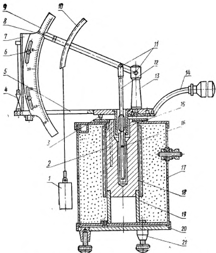
1 — груз; 2 — углубление для терморпары; 3 — опоры съемной части; 4 — отвес; 5 — станина; 6 — винты для крепления шкалы; 7 и 13 — стойки; 8 — рычаг; 9 — шкала; 10 — кулиса; 11 — штифты; 12 — штемпель; 14 — ручка съемной части аппарата; 15 — стаканчик; 16 — трубка со вставным донышком; 17 — кожух электропечи; 18 — толстостенный цилиндр электропечи с обмоткой из никромовой спирали; 19 — подставка под цилиндр; 20 — подставка; 21 — установочные винты.
