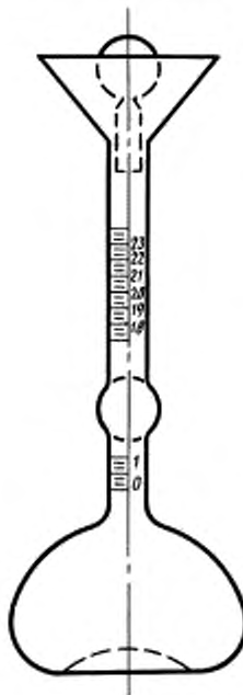
Прибор для определения плотности цемента
