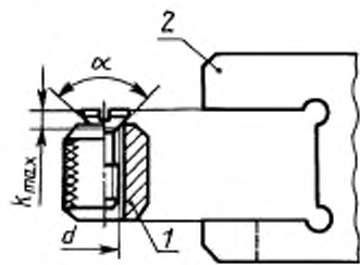
1 — втулка калибра; 2 — скоба калибра или индикатор
