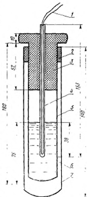
1—термометр; 2—кольцо из пенополистирола; 3—вкладыш из фторопласта; 4—чекол; 5—внутренняя пробирка; 6—смола; 7—внешняя пробирка. Черт. 2
