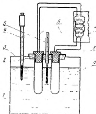
1 — теплоноситель—вода, 2—крышка термостата; 3—термостат; 4—контактный термометр; 5—ртутный термометр; 6—термопара; 7—потенциометр; 8—вкладыш из фторопласта, 9—наружная пробирка (см. черт. 2)
