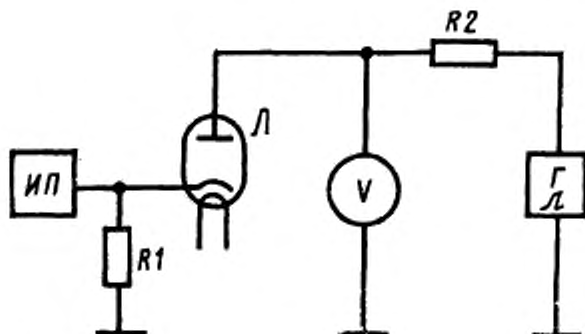
Л — испытываемая лампа; ИП — импульсный вольтметр или осциллограф; R1 — безындуктивный измерительный резистор; R2 — безындуктивный ограничительный резистор; V — импульсный вольтметр; ГЛ — генератор импульсов.
