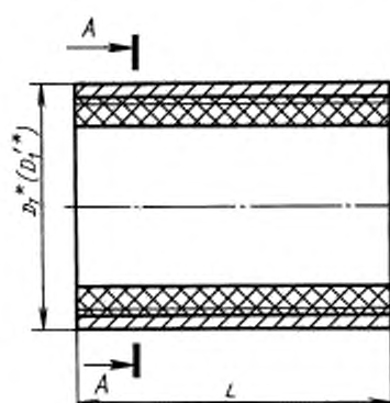
Подшипник типа I
