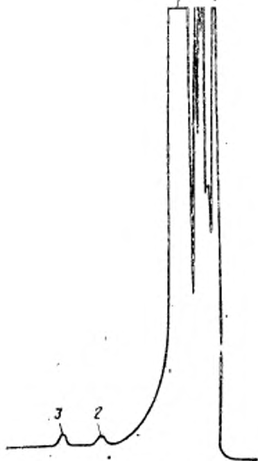
1—этилбензол; 2—диэтилбензол; 3—м-этил-изопропилбензол
