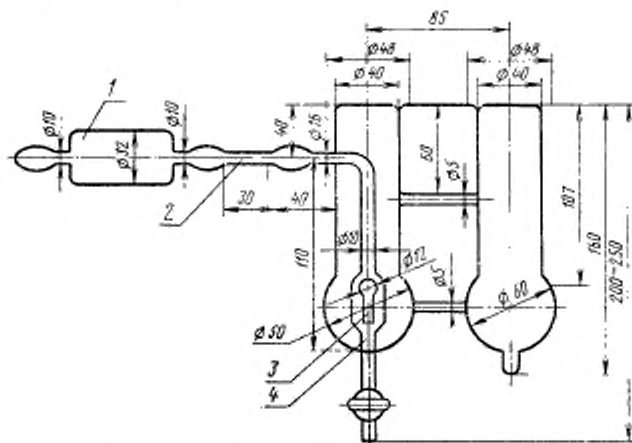
1—выселеватель; 2—резиновая трубка; 3—поплавок; 4—четыре отверстия Ø 1,5 мм
