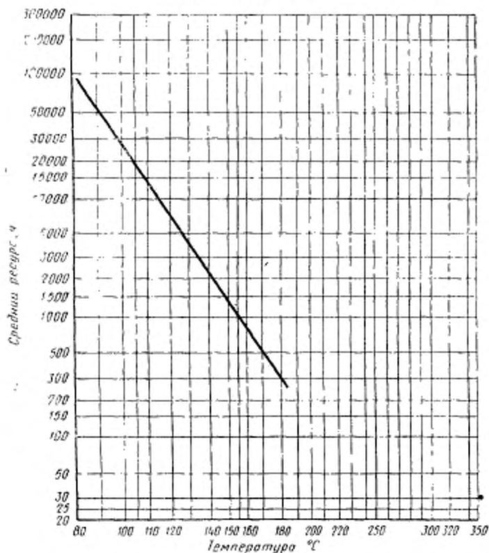
ГРАФИК ЗАВИСИМОСТИ СРЕДНЕГО РЕСУРСА ПРОВОДОВ ОТ ТЕМПЕРАТУРЫ
