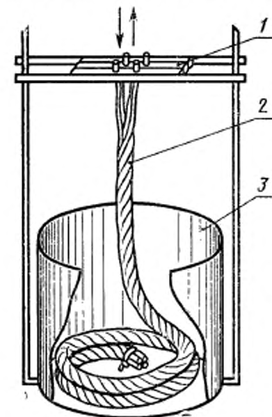
1—закрепляющие планки; 2—образец кабеля; 3—направляющий цилиндр
