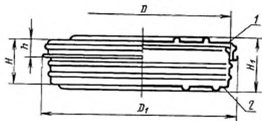
1 — крышка; 2 — корпус
