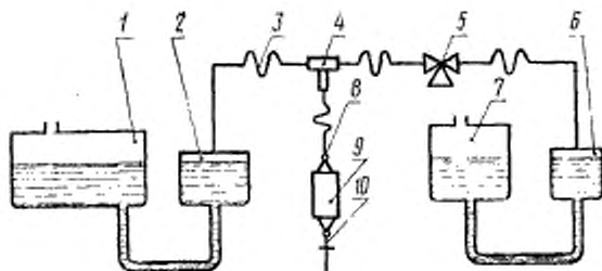
1, 2—подвижный и неподвижный сосуды образцового микроманометра; 3—резиновые трубки; 4—тройники; 5—трехходовый пробковый кран; 6, 7—неподвижный и подвижный сосуды поверяемого микроманометра; 9—сифонный пресс с кранами 8, 10
