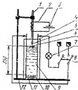
1—электромагнитный стержень; 2—обмотка стержня; 3—батарея; 4—цилиндрический сосуд; 5—шарик; 6—уровень клея; 7—лампа накаливания; 8—переключатель; 9—клеммы; 10—контактные штифты; 11—эбонитовая доска; 12—штатив.
