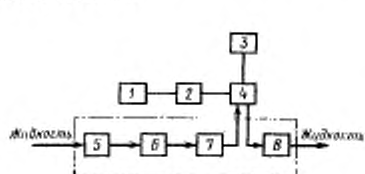
Блок измерения
