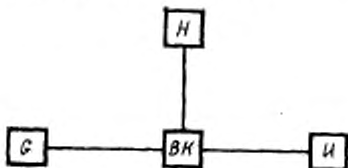
Г—генератор; Н—нагрузка; ВК—выходной контур; И—индикаторное устройство.
