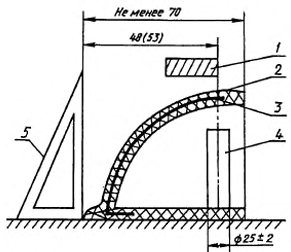
1 — боек; 2 — носок; 3 — ударозащитный поднос; 4 — пластилиновый столбик; 5 — угольник
