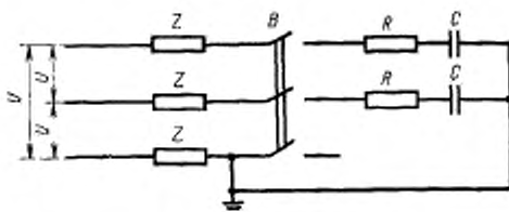
U —испытательное напряжение; Z —полное сопротивление источника питания; B —выключатель нагрузки; R —активное сопротивление; C —емкость.
