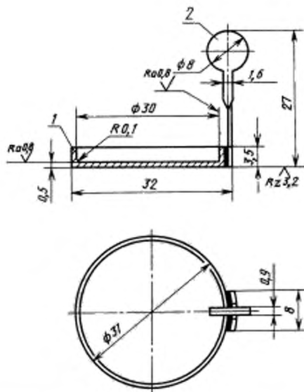
1 — чашка; 2 — ручка
