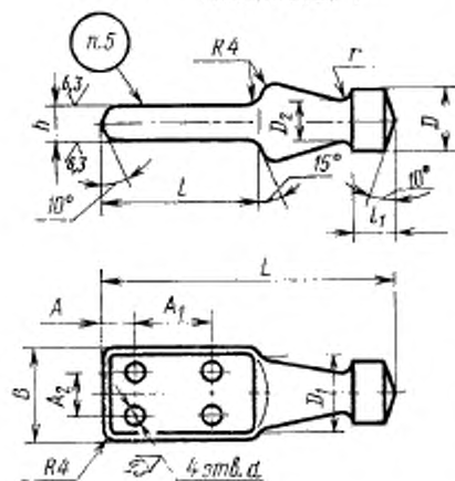
Исполнение 1
