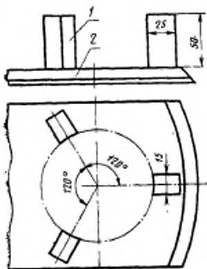
1—ограничитель; 2—подставка
