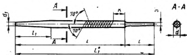
Круглые напильники с нарезанными зубьями
