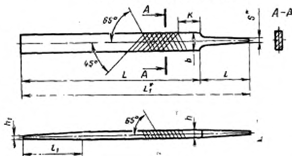
Плоские тупоносые напильники
