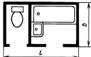
Правые варианты исполнения кабин
