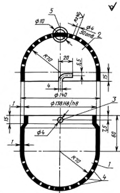
Контейнер для насыщения заполнителя водой
