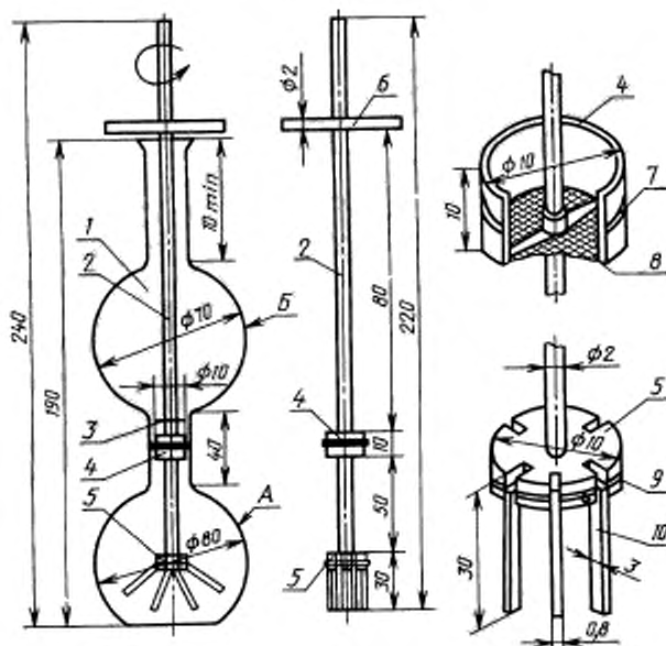
1 — основная (А) и дополнительная (Б) емкости двойной колбы; 2 — шток; 3 — метка; 4 — поршень; 5 — поршень-мешалка; 6 — перекладина; 7 — уплотнительное кольцо; 8 — сетка № 063; 9 — ободок из проволоки диаметром 1 мм; 10 — лопасти
