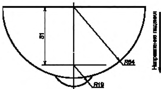
Рисунок Т.1 — Модель головы
