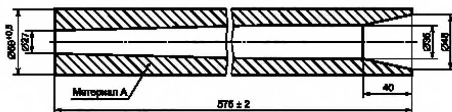
Рисунок Е.12 — Полиуретановая трубка
