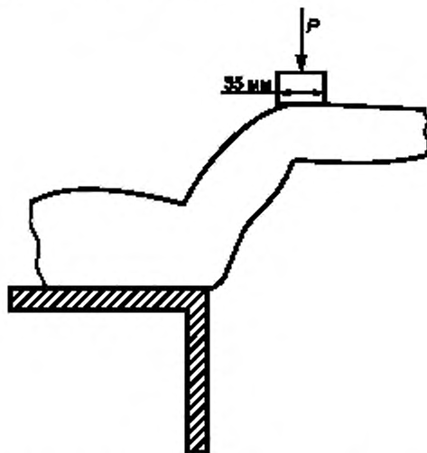
Рисунок И.12 — Калибровка жесткости сочленения ноги
