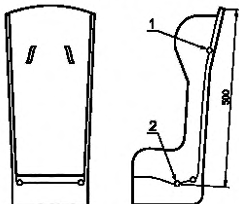
Рисунок Н.1 — Места крепления
