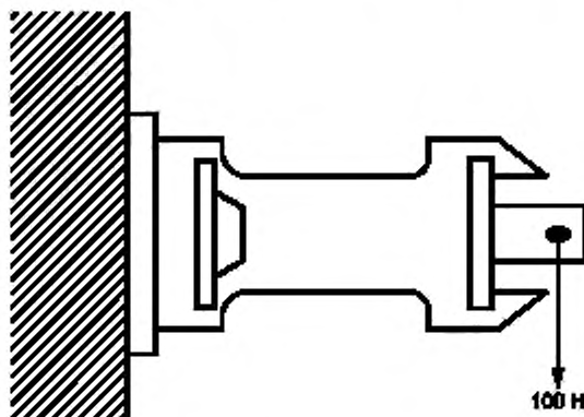
Рисунок И.16 — Монтаж элемента шеи в комплекте
