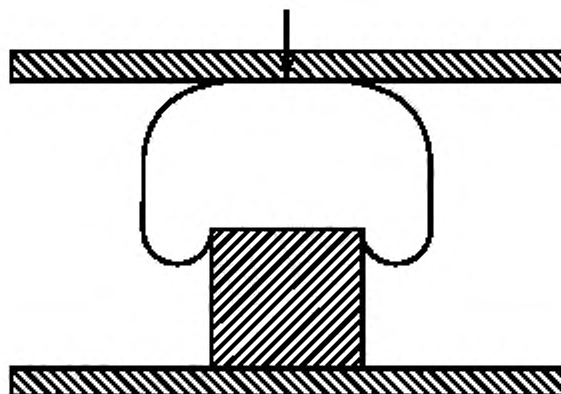
Рисунок И.9 — Калибровка полости живота
