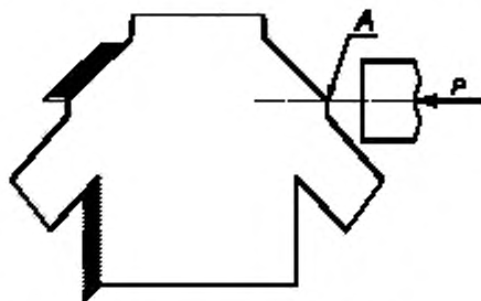
Рисунок И.11 — Калибровка жесткости плечевого сустава
