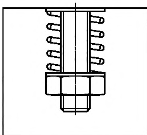
Рисунок И.8 — Регулирование поясничного троса
