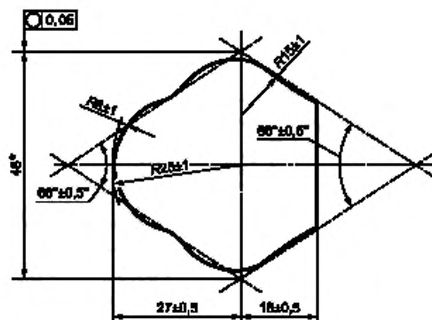
Рисунок Е.9 — Основные размеры овального наконечника стопорного устройства
