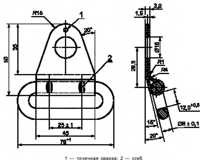
Поверхность изделия хромированная. Рисунок П.4 — Прикрепляемый к стойке хомут
