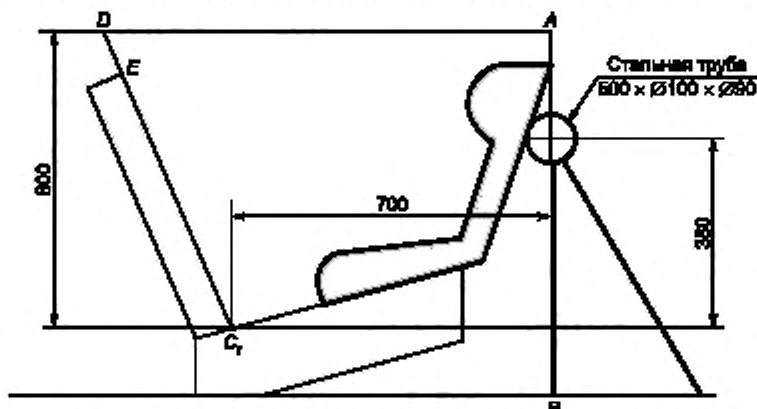
Рисунок 2 — Схема испытания детского удерживающего устройства, обращенного назад
