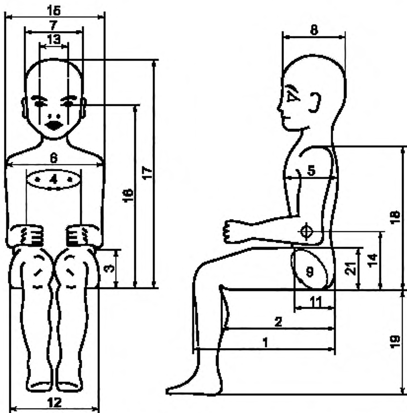
Рисунок И.1 — Основные размеры манекенов
