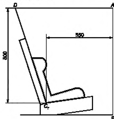
Рисунок 1 — Схема испытания детского удерживающего устройства, обращенного вперед
