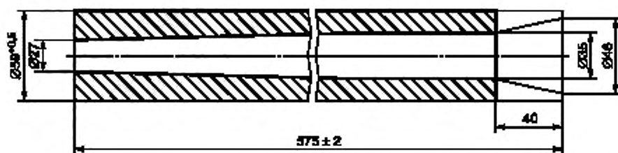
Рисунок Е.7 — Полиуретановая трубка из материала А
