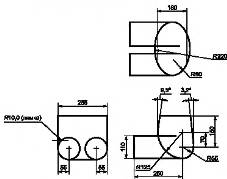
Рисунок Ш.1 — Манекен Р10 в разрезе
