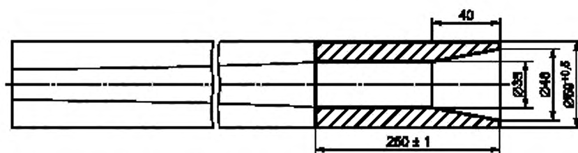
Рисунок Е.8 — Полиуретановая трубка из материала В
