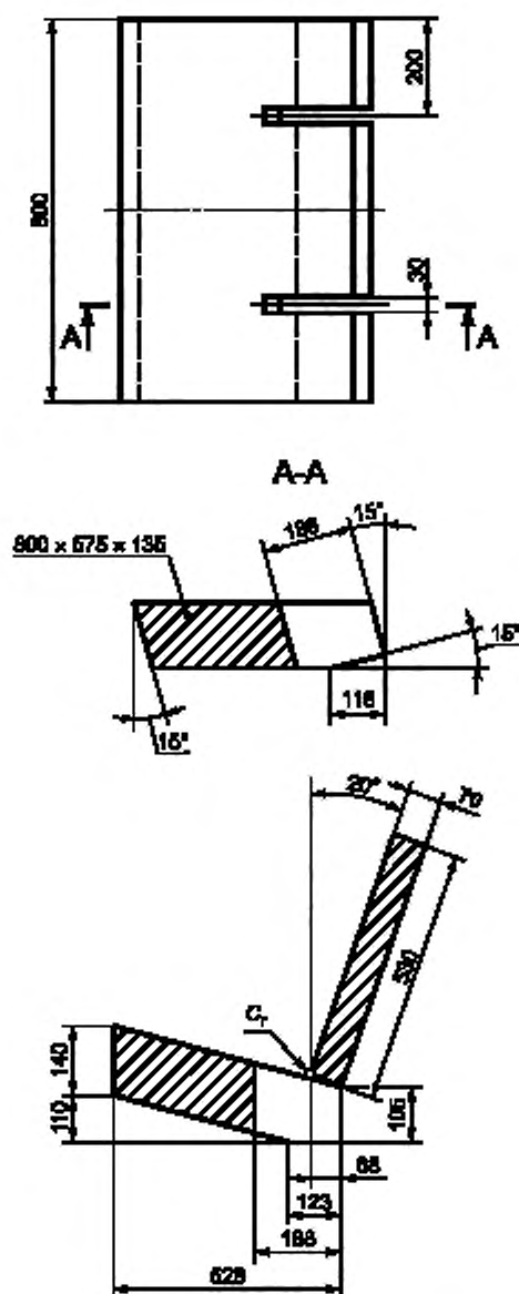
Рисунок Е.2 — Размеры сиденья и подушек сиденья
