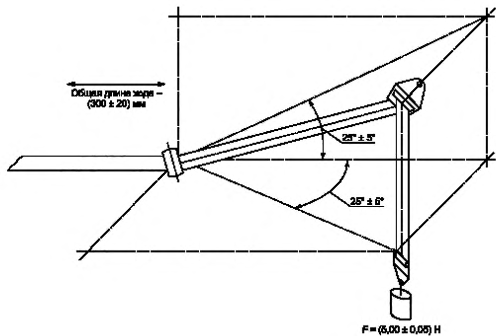
Рисунок Д.4 — Испытание с направляющим устройством
