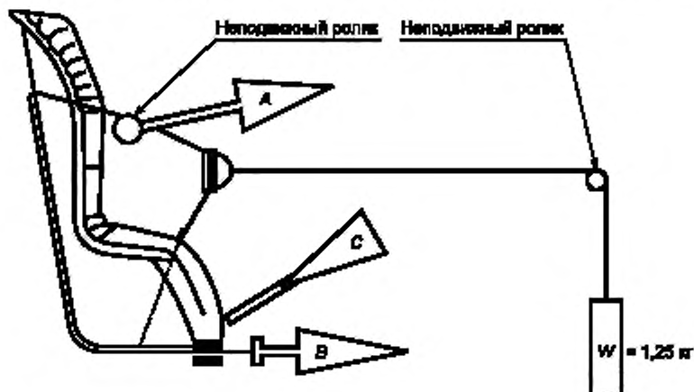
Рисунок X.1 — Схема испытательного устройства
