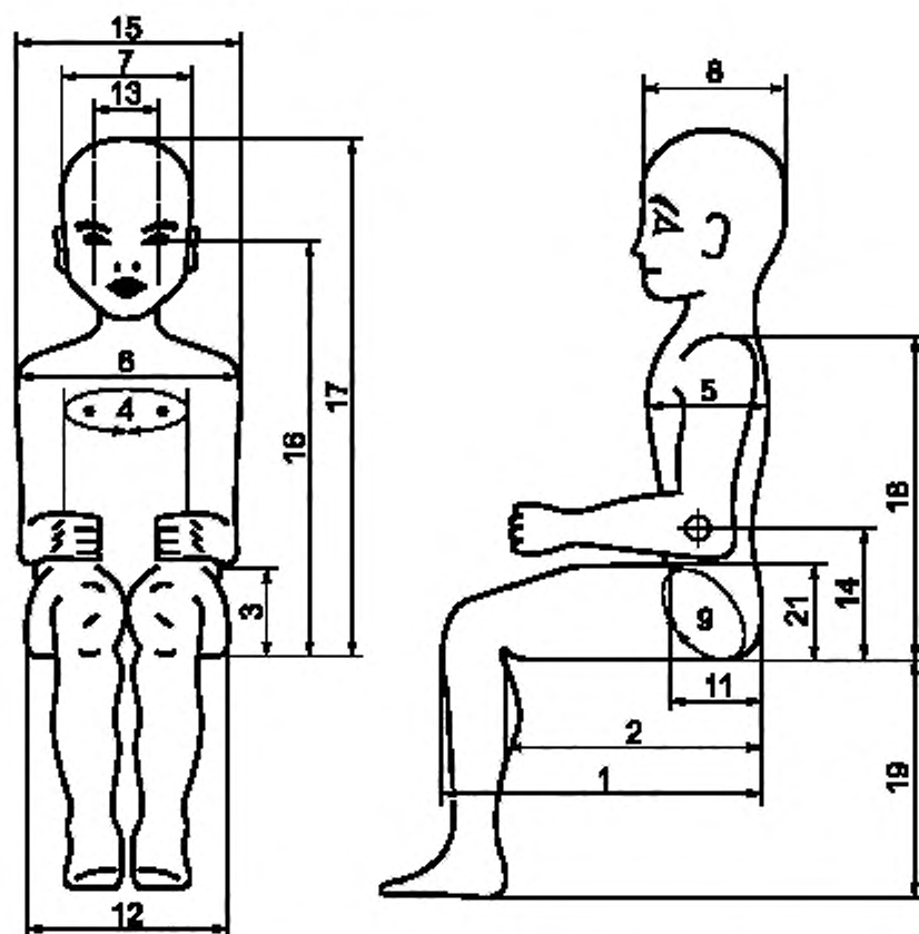
Рисунок И.13 — Основные размеры манекена 18-месячного ребенка
