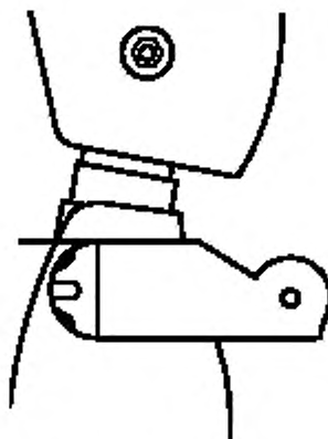
Рисунок И.6 — Регулирование плечевых сочленений
