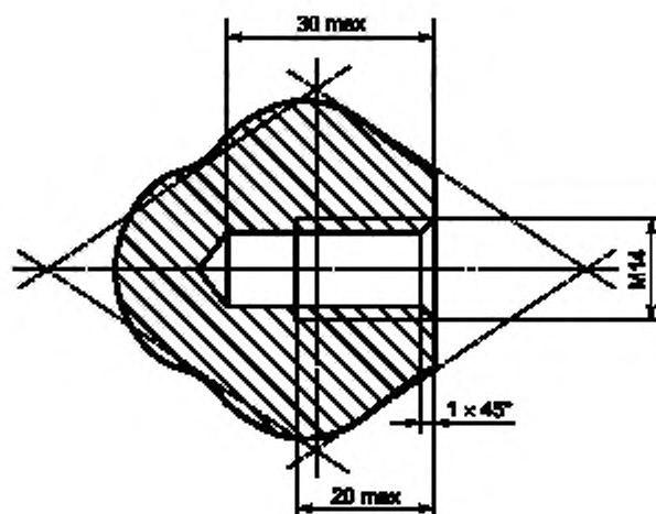
Рисунок Е.10 — Дополнительные размеры овального наконечника стопорного устройства
