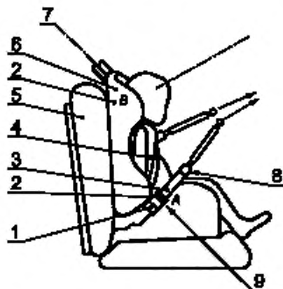
1 — пряжка/язычок; 2 — зажим; 3 — поясной ремень; 4 — диагональный ремень; 5 — испытательное сиденье типа ECE 44; 6 — детское сиденье; 7 — втягивающее устройство; 8 — D-образное кольцо; 9 — место проверки на проскальзывание
