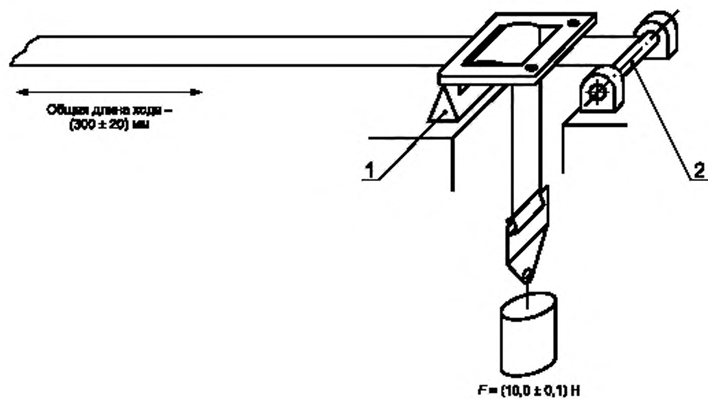
Рисунок Д.2 — Схема испытания В
