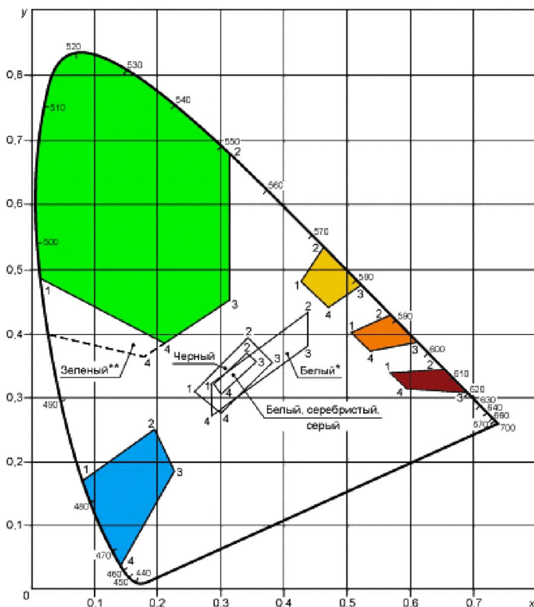
Рисунок 2 — График цветковых областей для знаков с внутренним и внешним освещением
