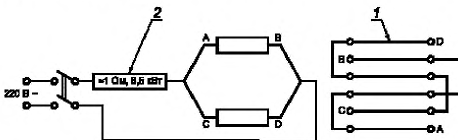
1 — стержень из карбида кремния; 2 — добавочное сопротивление
