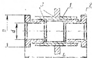
1 — гнездо; 2 — нажимная гайка исполнения 1; 3 — шайба
