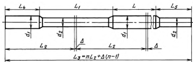
Размеры, мм
