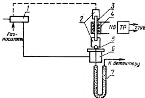
1—кран-дозатор; 2—соединительная трубка резиновая; 3—концентратор; 4—тер- мометр; 5—инъекционная игла; 6—испа- ритель; 7—хроматографическая колонка
