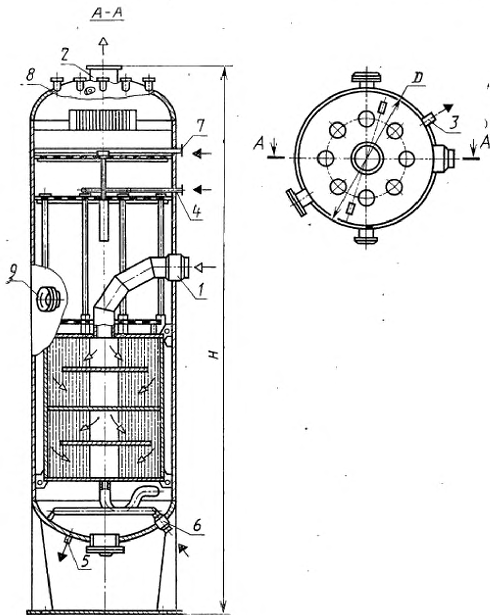
1—вход греющего пара; 2—выход вторичного пара; 3—выход конденсата; 4—вход промывочной питательной воды; 5—продувка; 6—вход питательной воды; 7—вход промывочного конденсата; 8—присоединение к предохранительному клапану; 9—люк.
